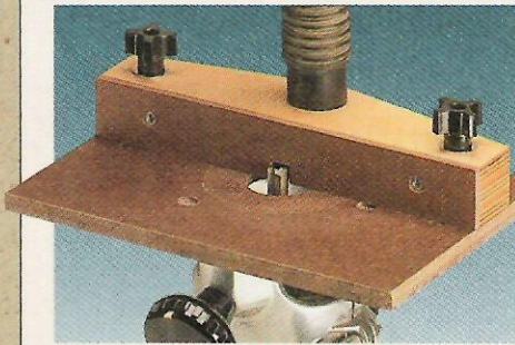
EDGE GUIDE
